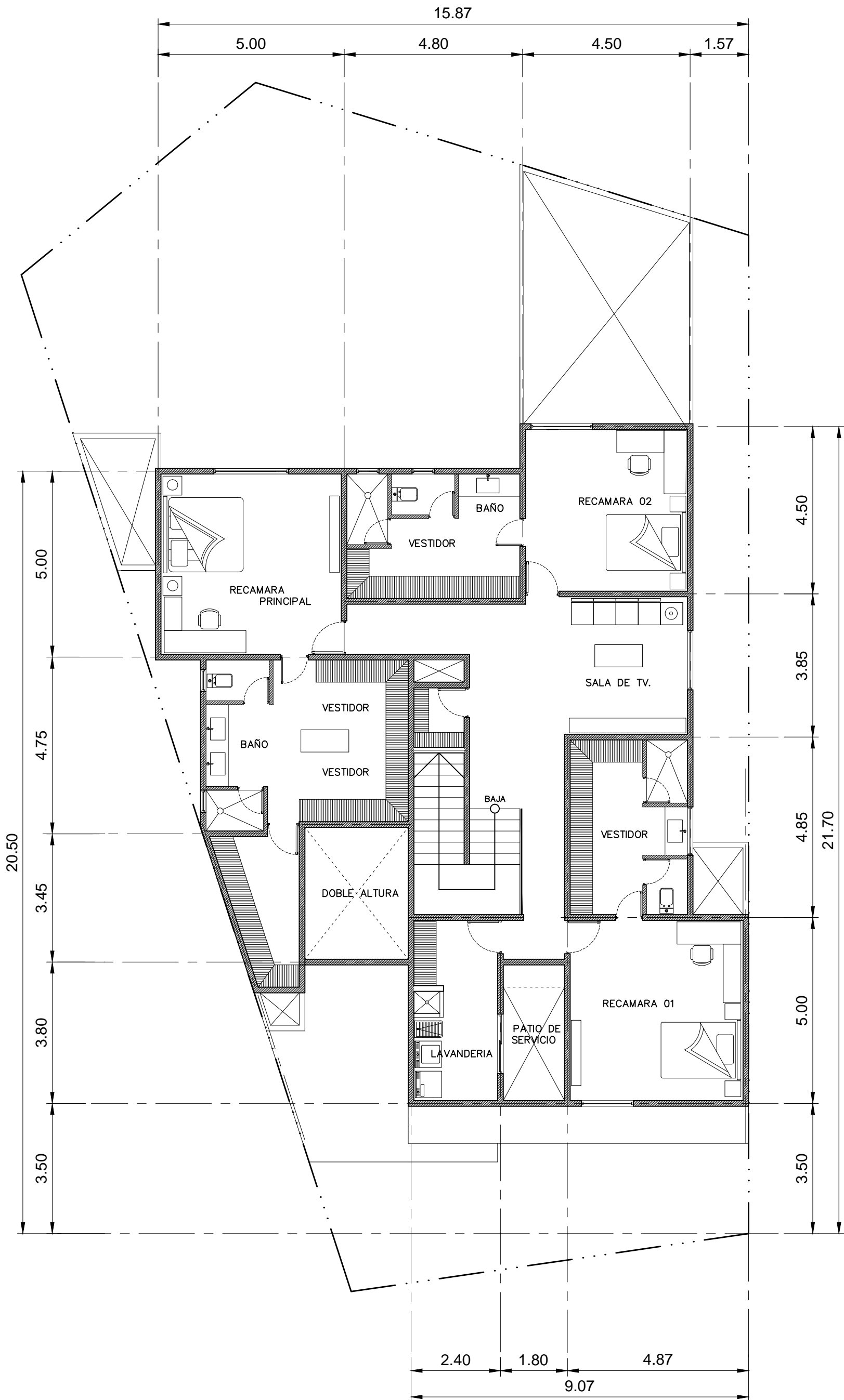
PLANTA ALTA ESC 1:100
