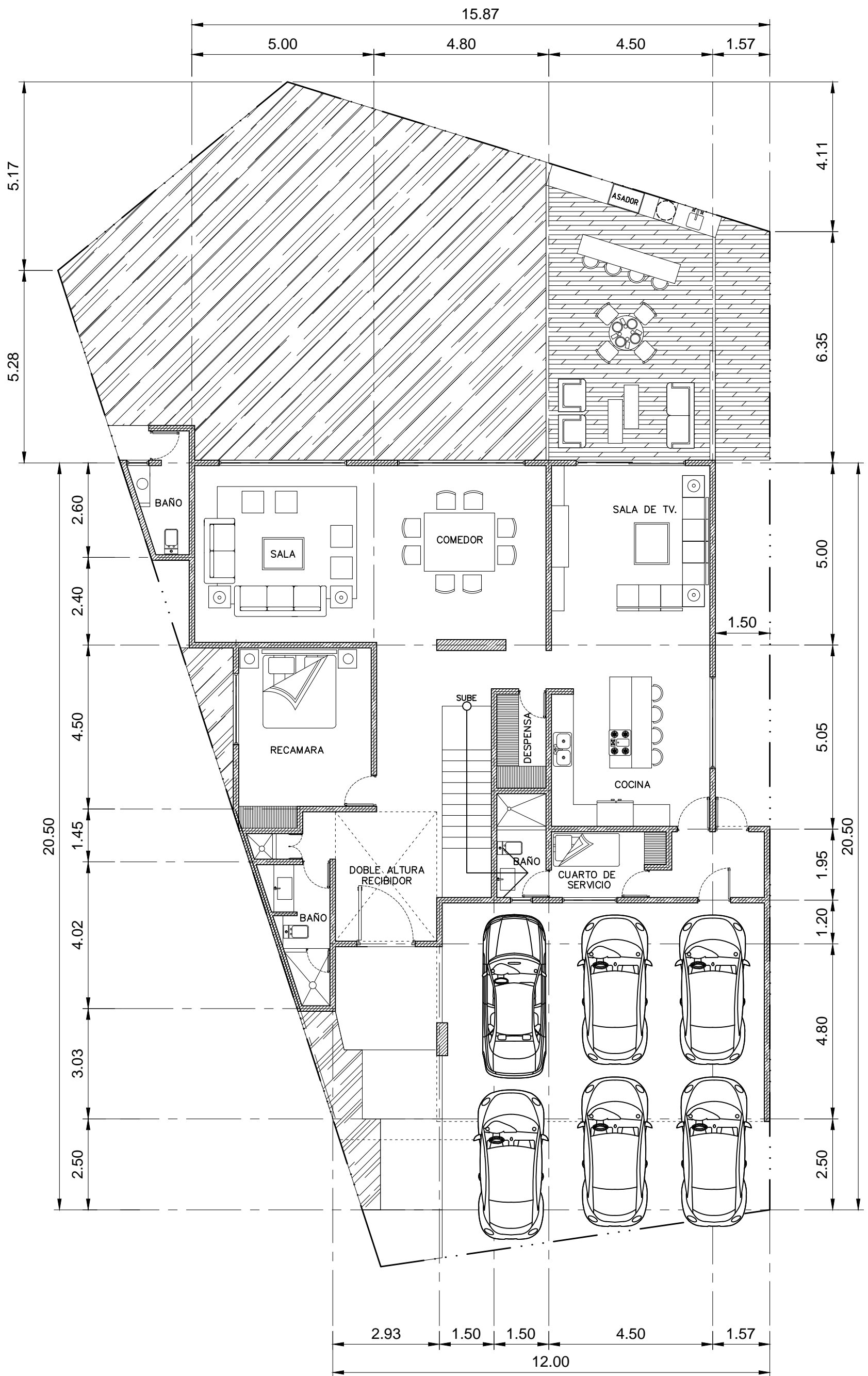
PLANTA BAJA
